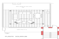
PLANTA SOLARIUM SUP. UTIL : 59,00 M2. SUP. CONSTRUIDA: 70,00 M2.
