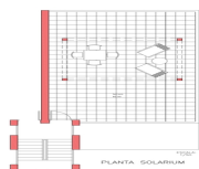
PLANTA SOLARIUM SUP. UTIL : 50,00 M2. SUP. CONSTRUIDA: 72,30 M2. SUP. DE TERRAZA DESEO : 11,00 M2. SUP. DE CUBIERTA : 60,00 M2.
